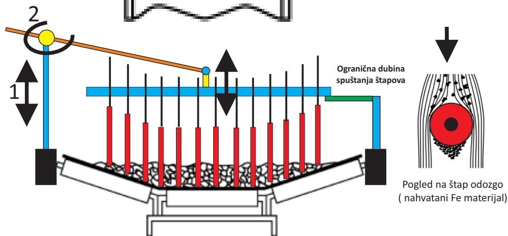
Raspored štapova na transportnoj traci (PRESEK)
